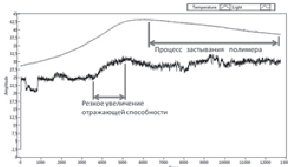
Графики температуры и освещенности в процессе получения полимера
