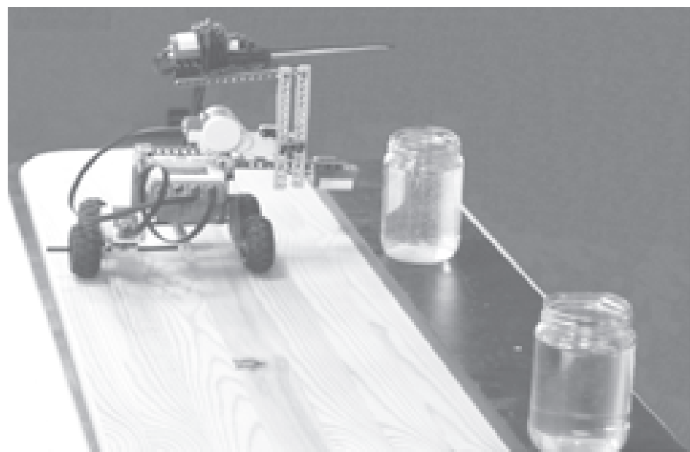
Робот с датчиком температуры Vernier
