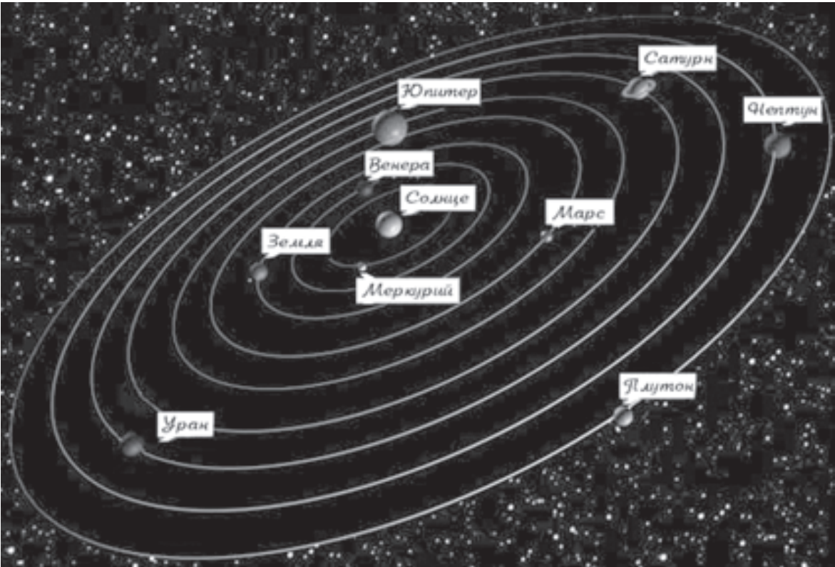
Схема Солнечной системы
